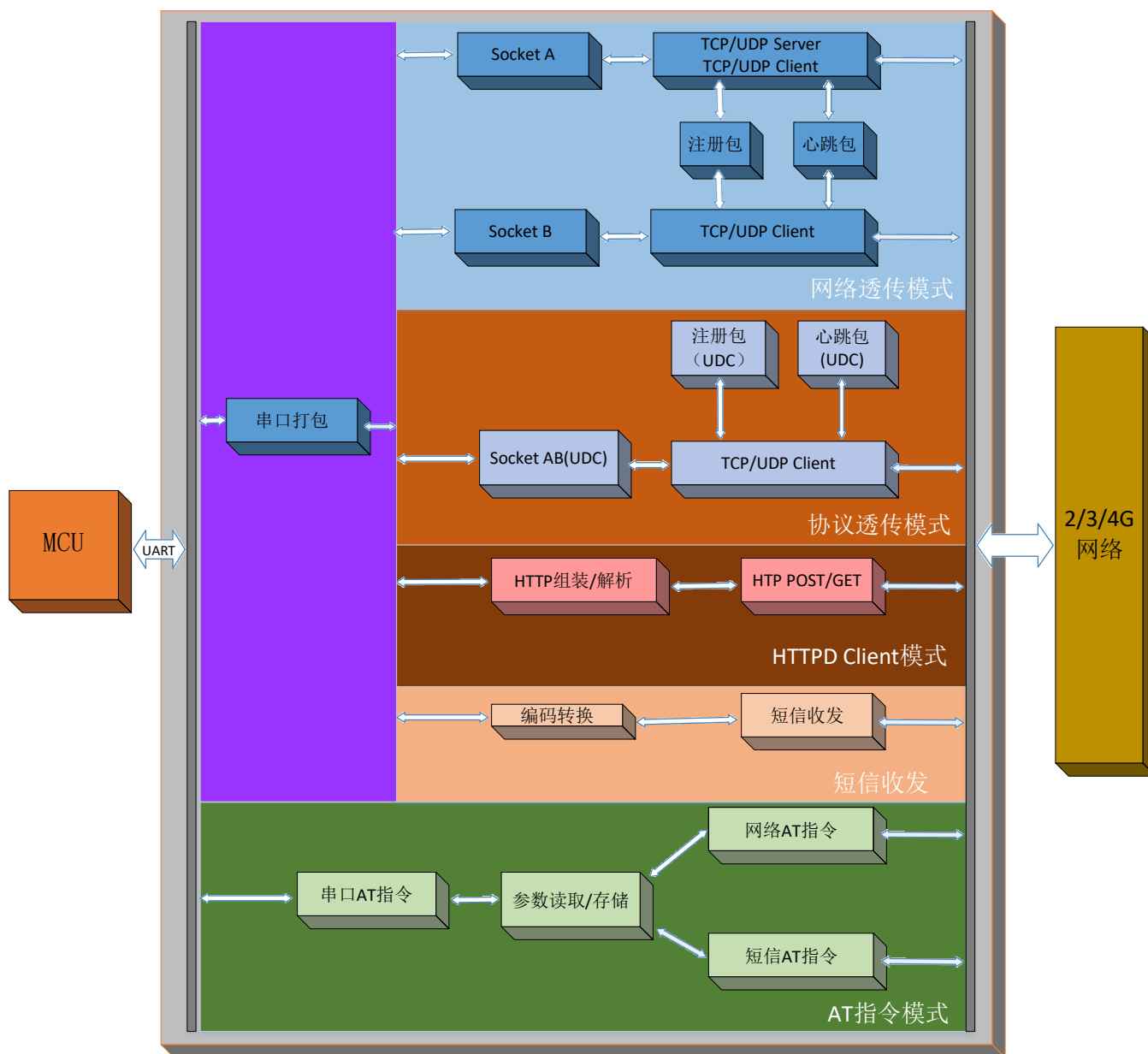
图 1 功能框图
