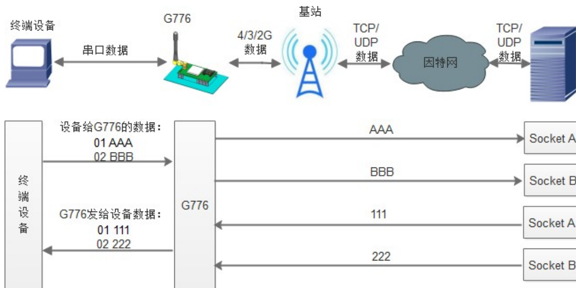
图 16 套接字分发协议示意图
