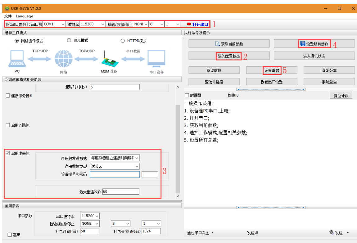
设置软件示意图：
