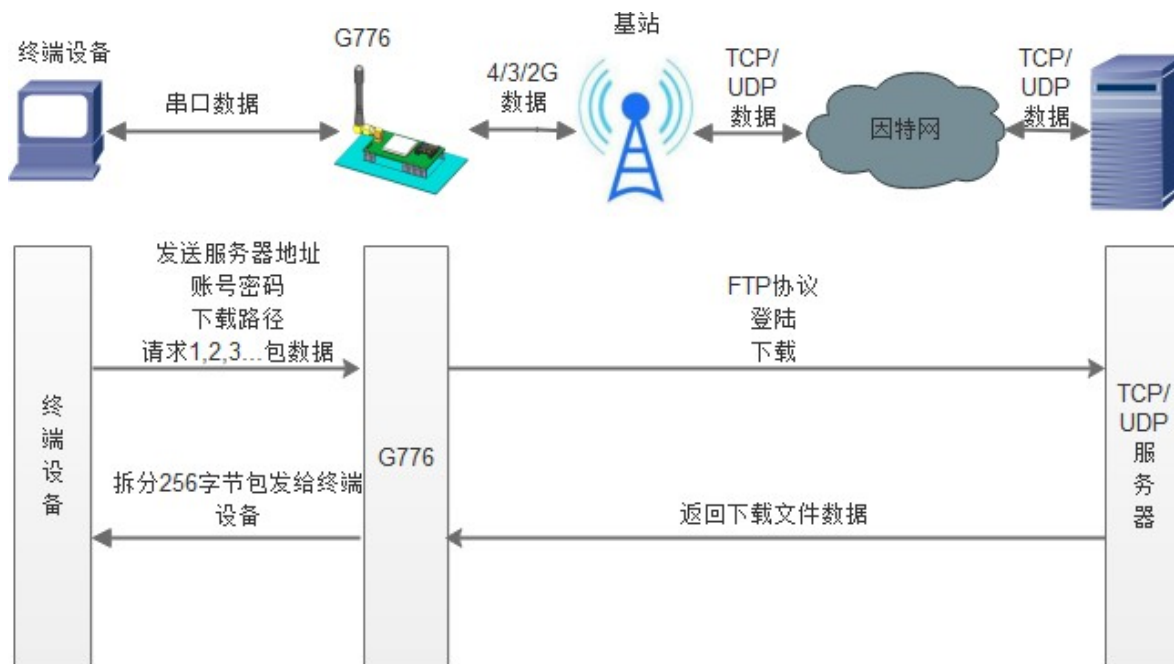
图 17 FTP 他升级协议示意图
