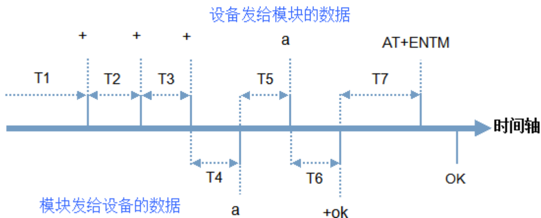
图 20 模式切换时序图
