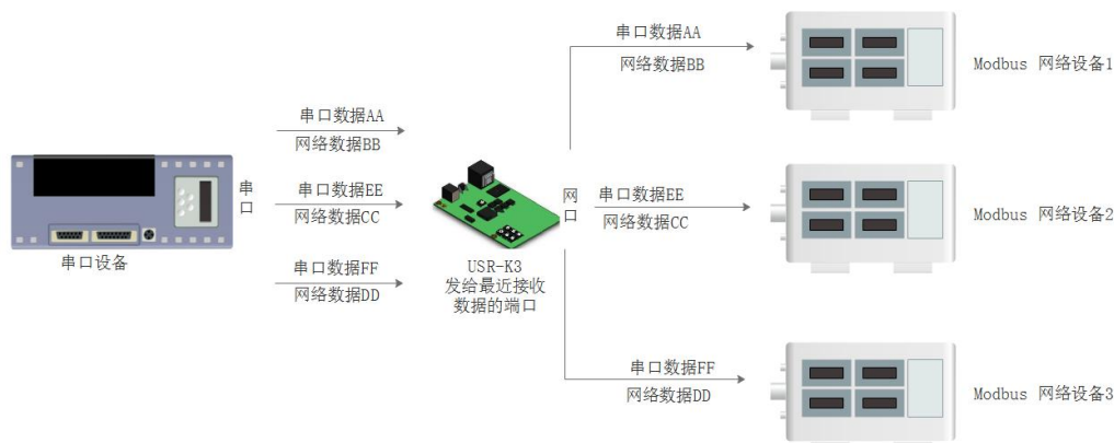
图 46 Modbus TCP
