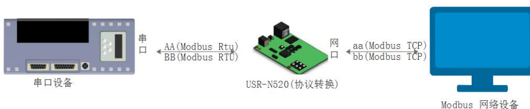
图 39 Modbus TCP
