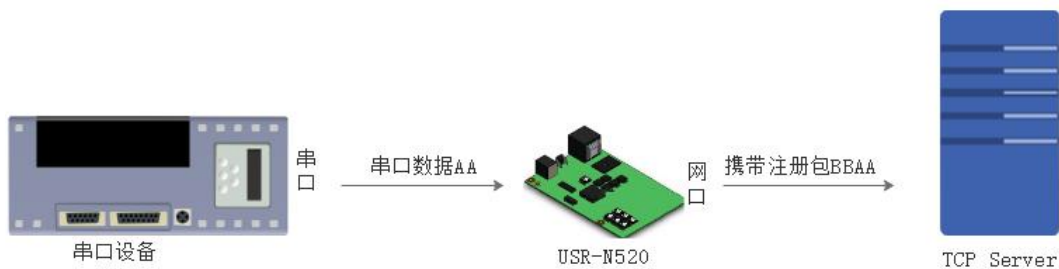
图 52 数据携带
