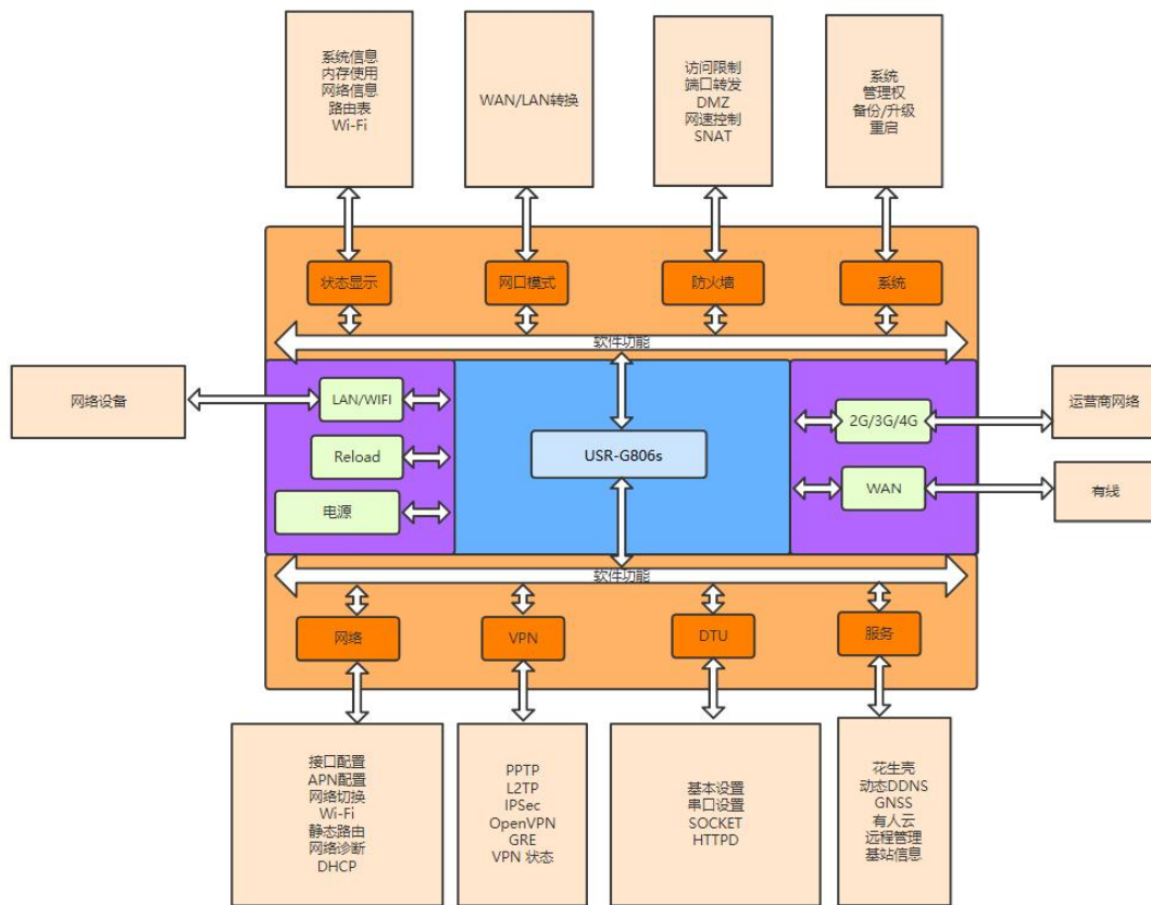
图 3 功能框图
